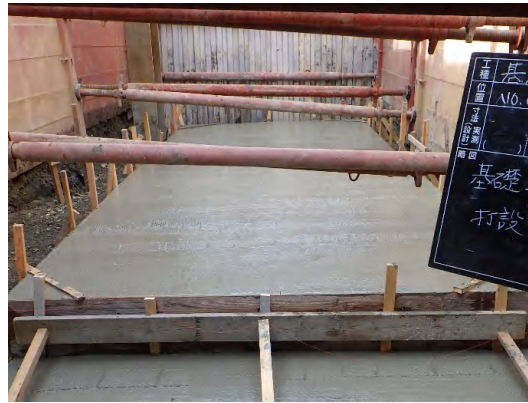
基礎工(コンクリート打設)状況
