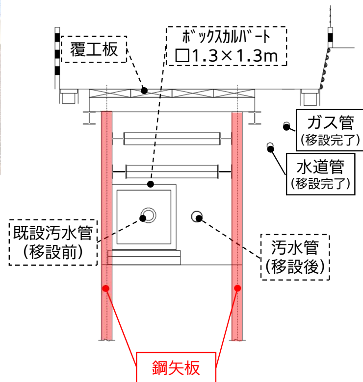
仮設土留(ア-オーガ)施工状況
