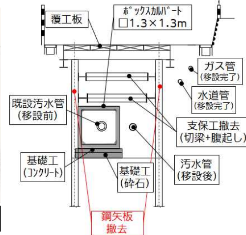
ボックスカルバート(内部)布設完了
