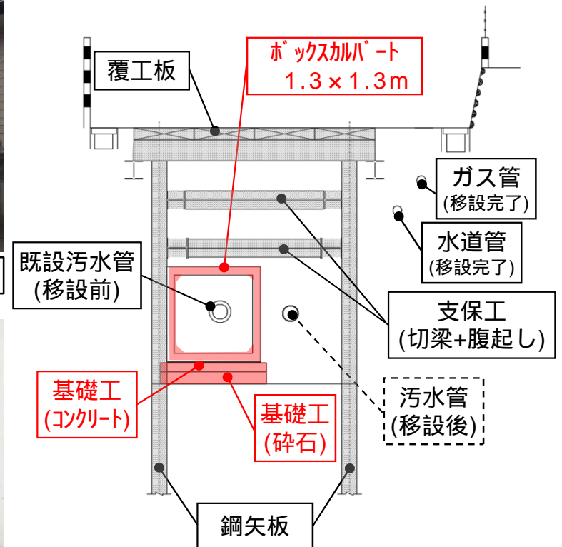
ボックスカルバート布設状況
