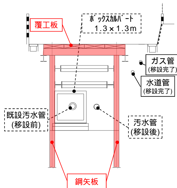
仮設土留(鋼矢板)施工完了状況
