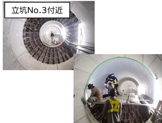
鋼製セグメント二次覆工状況
