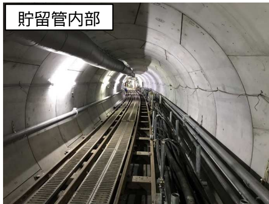
シールド掘進機による初期掘進完了
