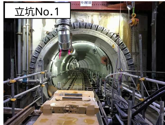
仮セグメント撤去完了
