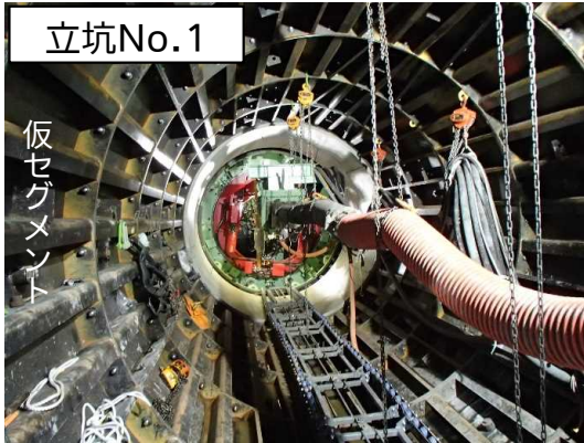
シールド掘進機※による掘進状況
