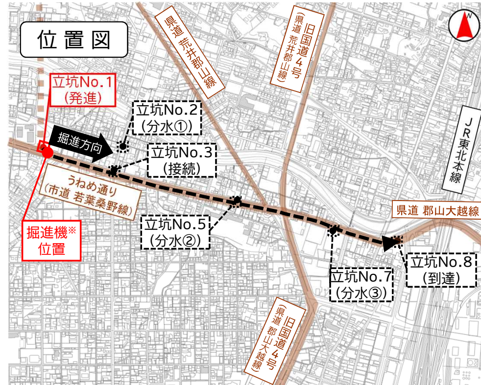
シールド掘進機※による掘進状況
