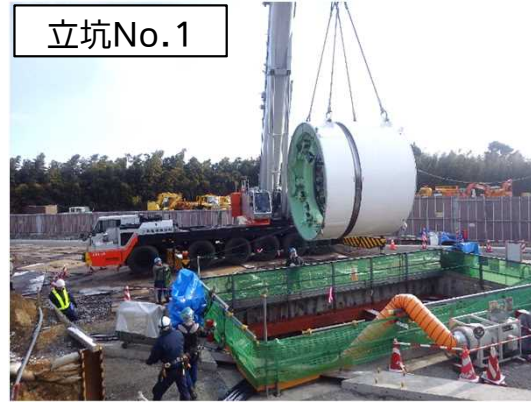
シールド掘進機分割搬入状況
