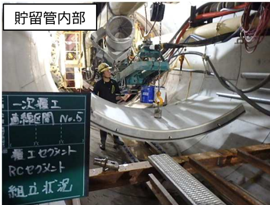
シールド掘進機による掘進状況(セグメント設置)
