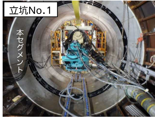
セグメント※設置状況
