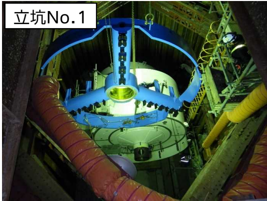
シールド掘進機搬入・設置状況
