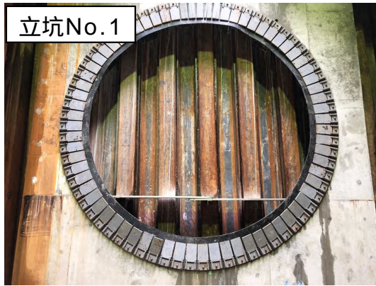
坑口施工(コンクリート打設完了)状況
