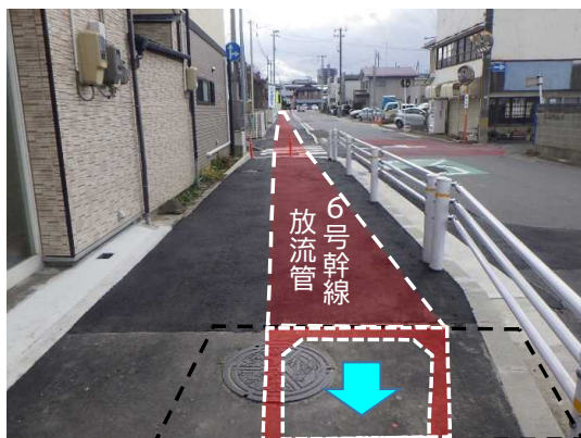
舗装仮復旧状況(下流側より上流側へ)
