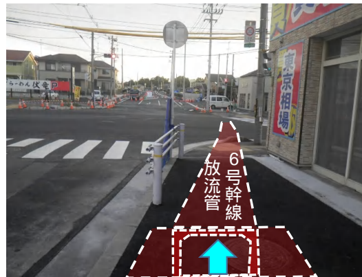
舗装本復旧状況(上流側から下流側を望む)
