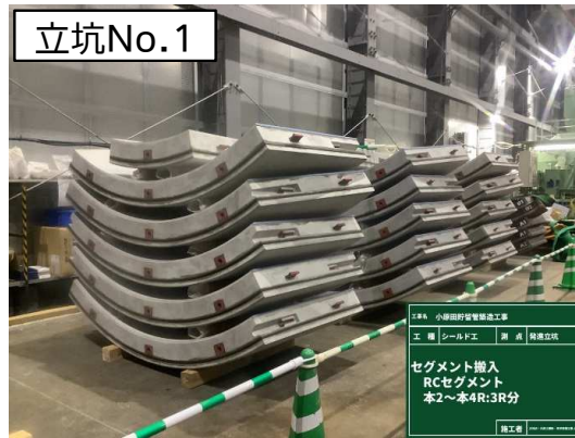
セグメント搬入保管状況(仮設防音ハウス内)
