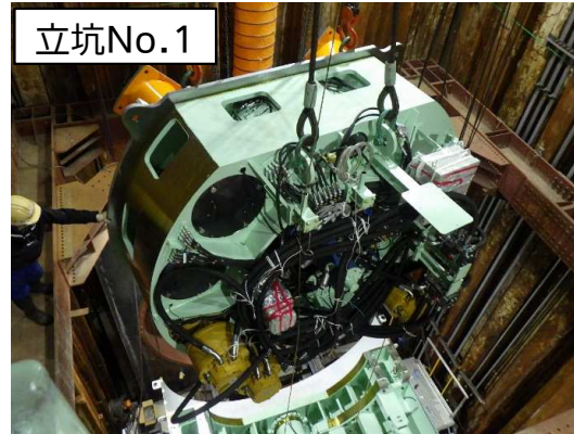
シールド掘進機投入・組立状況
