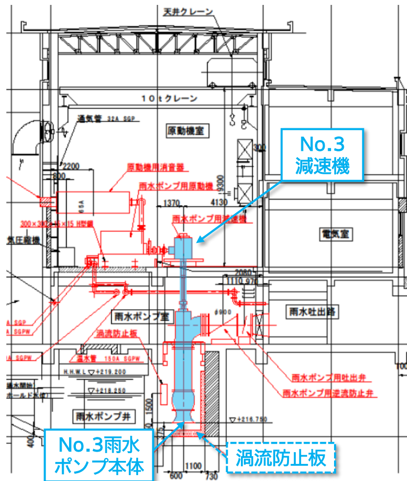
断面図(1階・地下1階・地下2階)
