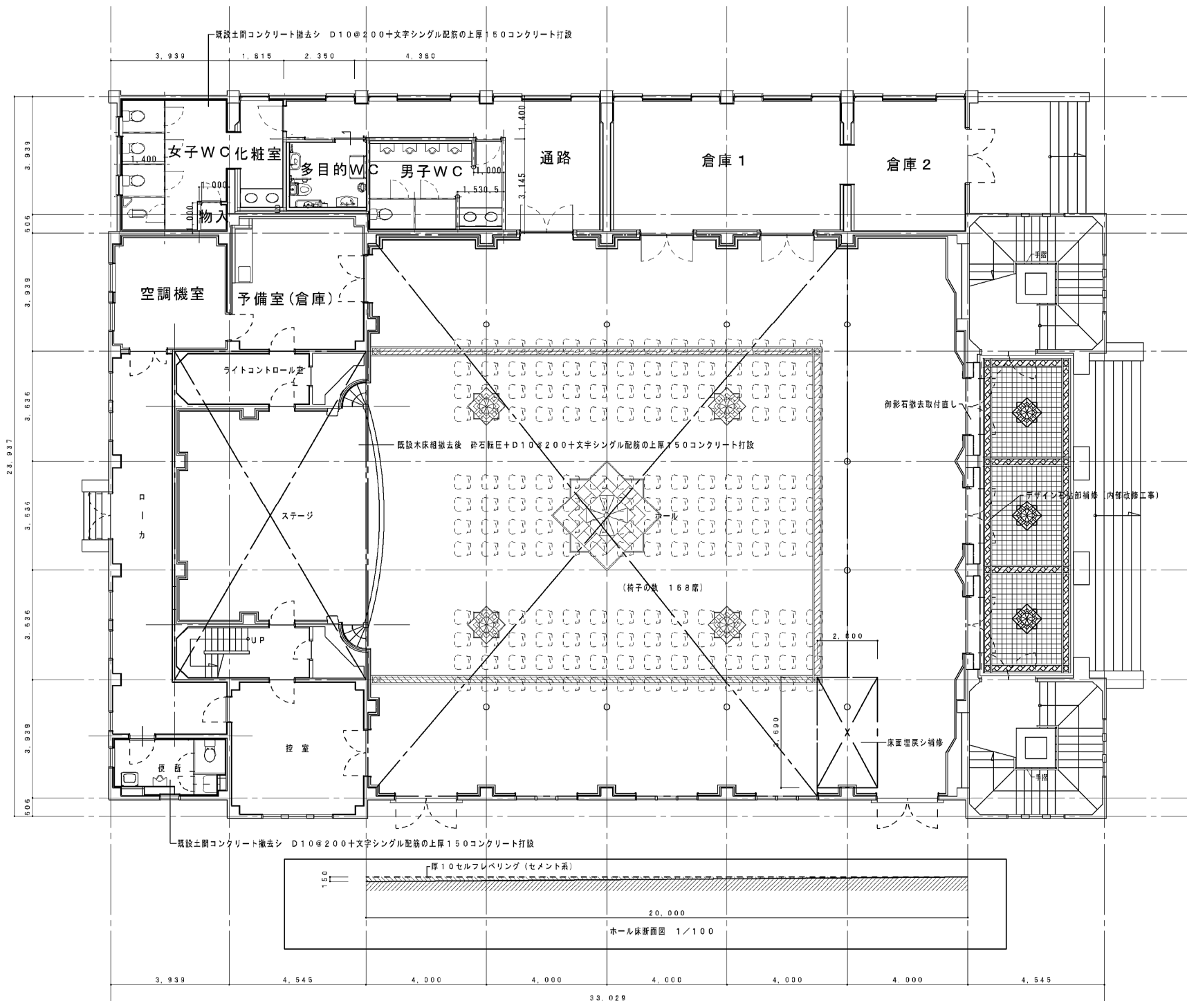
1階平面図 1/100
