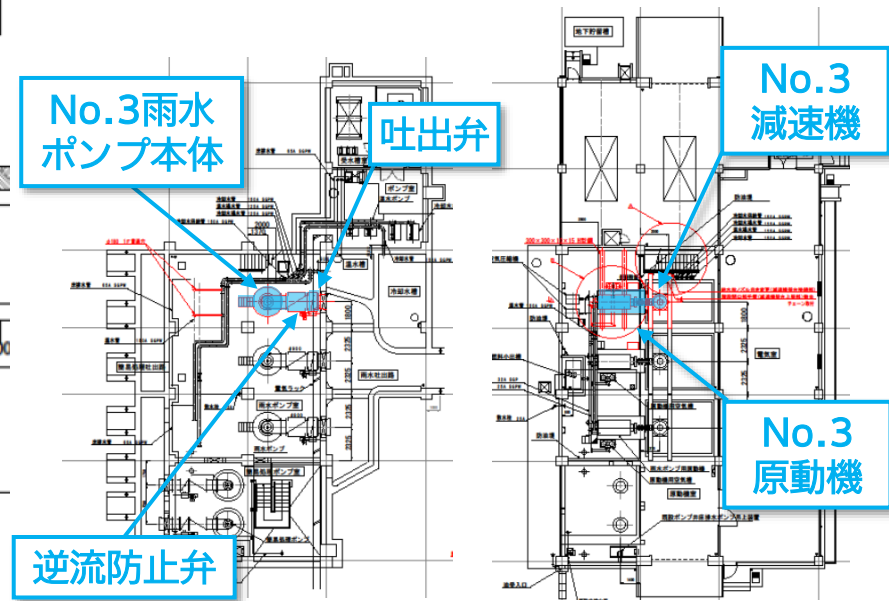
平面図(地下1階)
