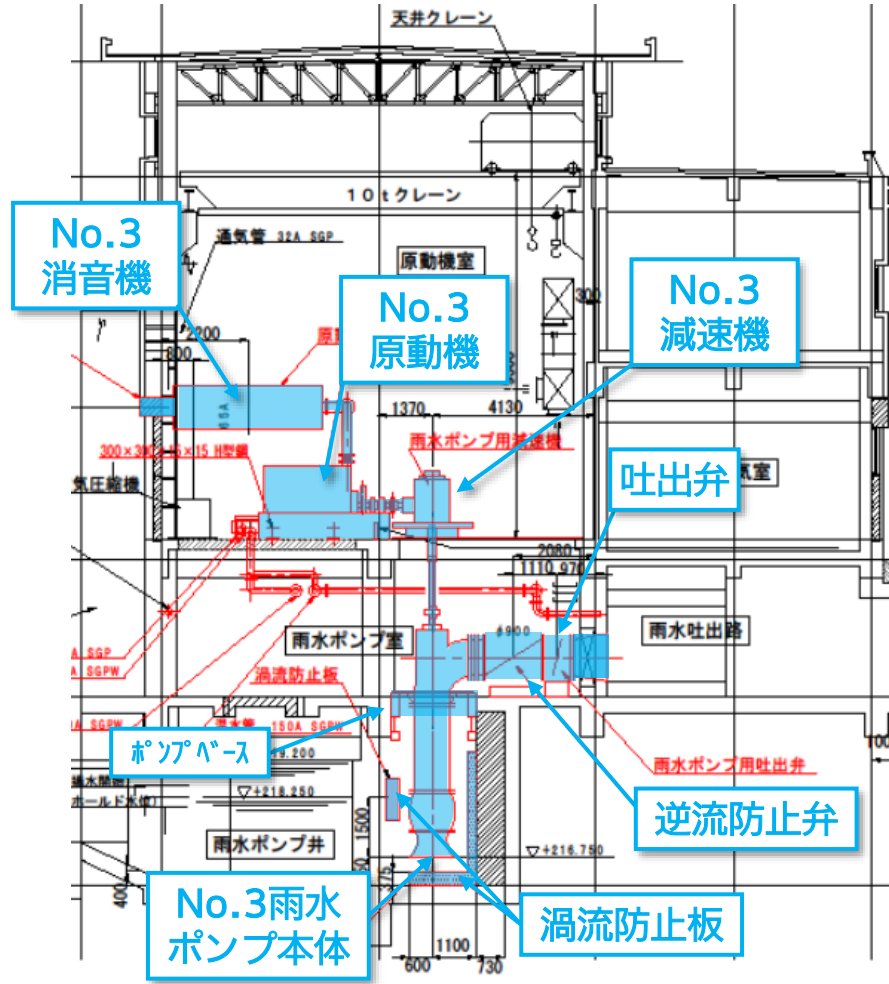
断面図(1階・地下1階・地下2階)
