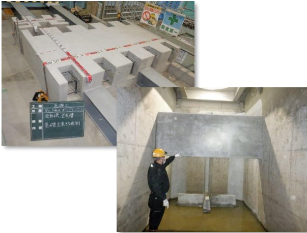
雨水ポンプ用原動機基礎工、渦流防止板築造状況
