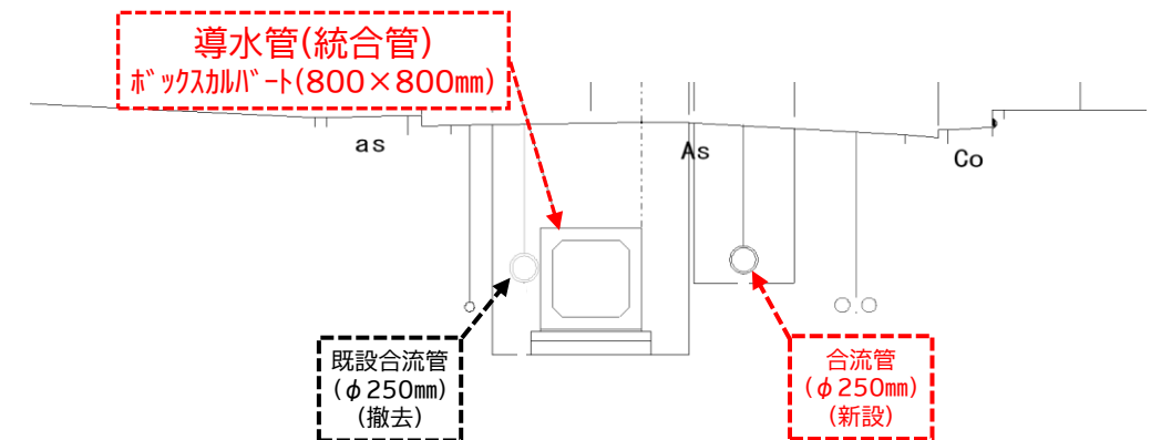
計画断面図
