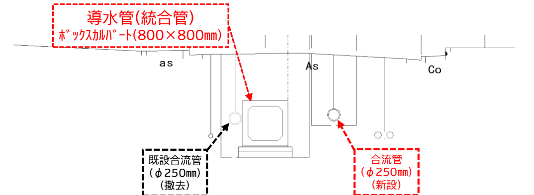
計画断面図
