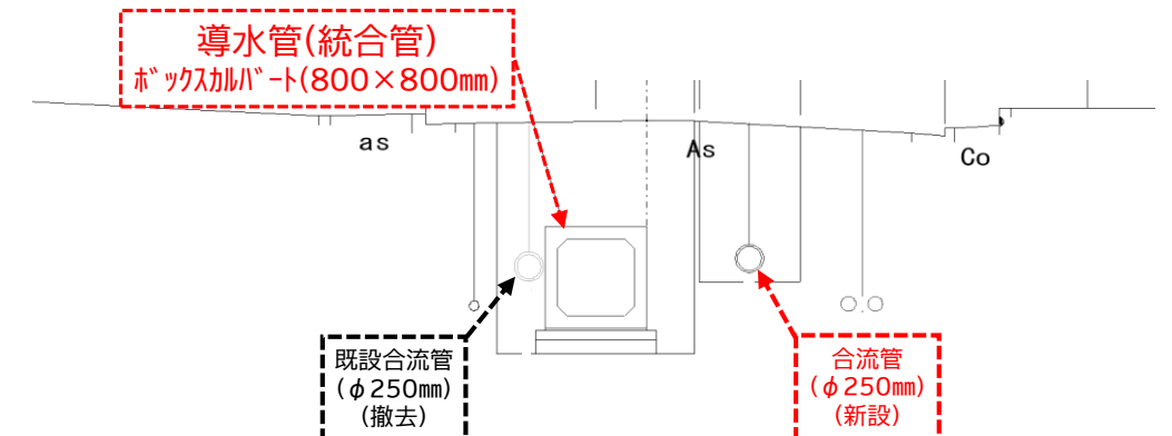
計画断面図
