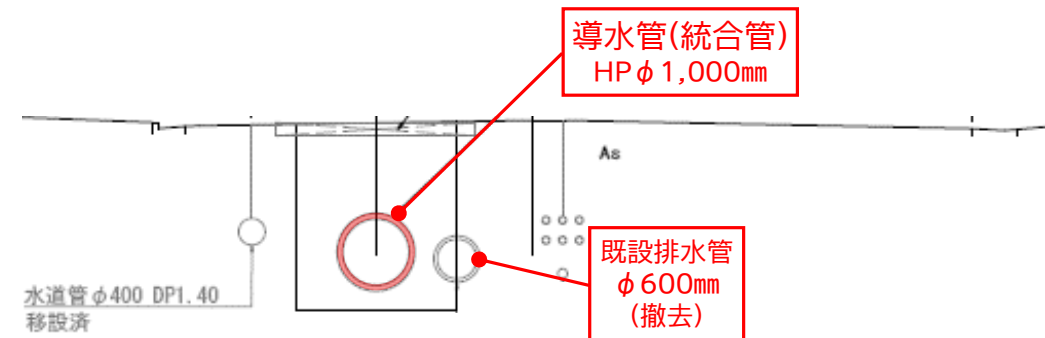
計画断面図
