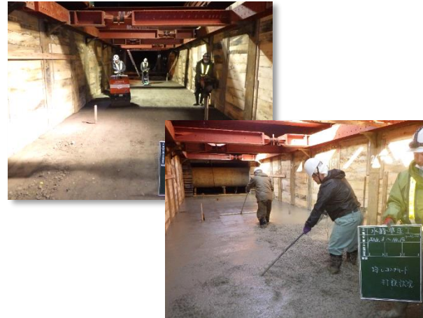
基礎工(砕石・コンクリート打設)状況
