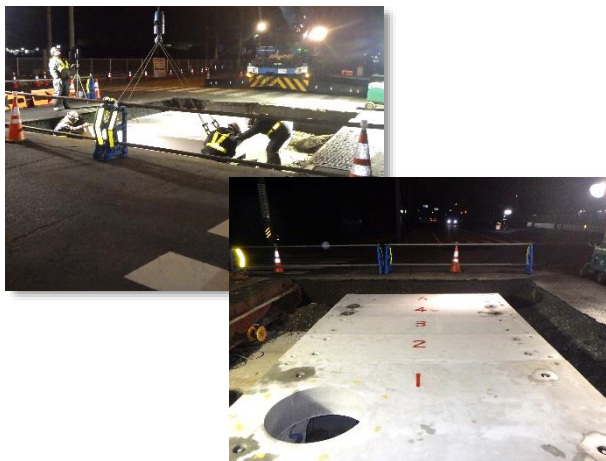
No.3特殊人孔築造(床版据付)状況
