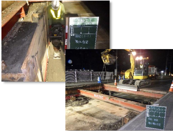
埋戻し・転圧、覆工板受桁撤去状況
