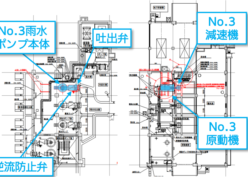
平面図(地下1階)
