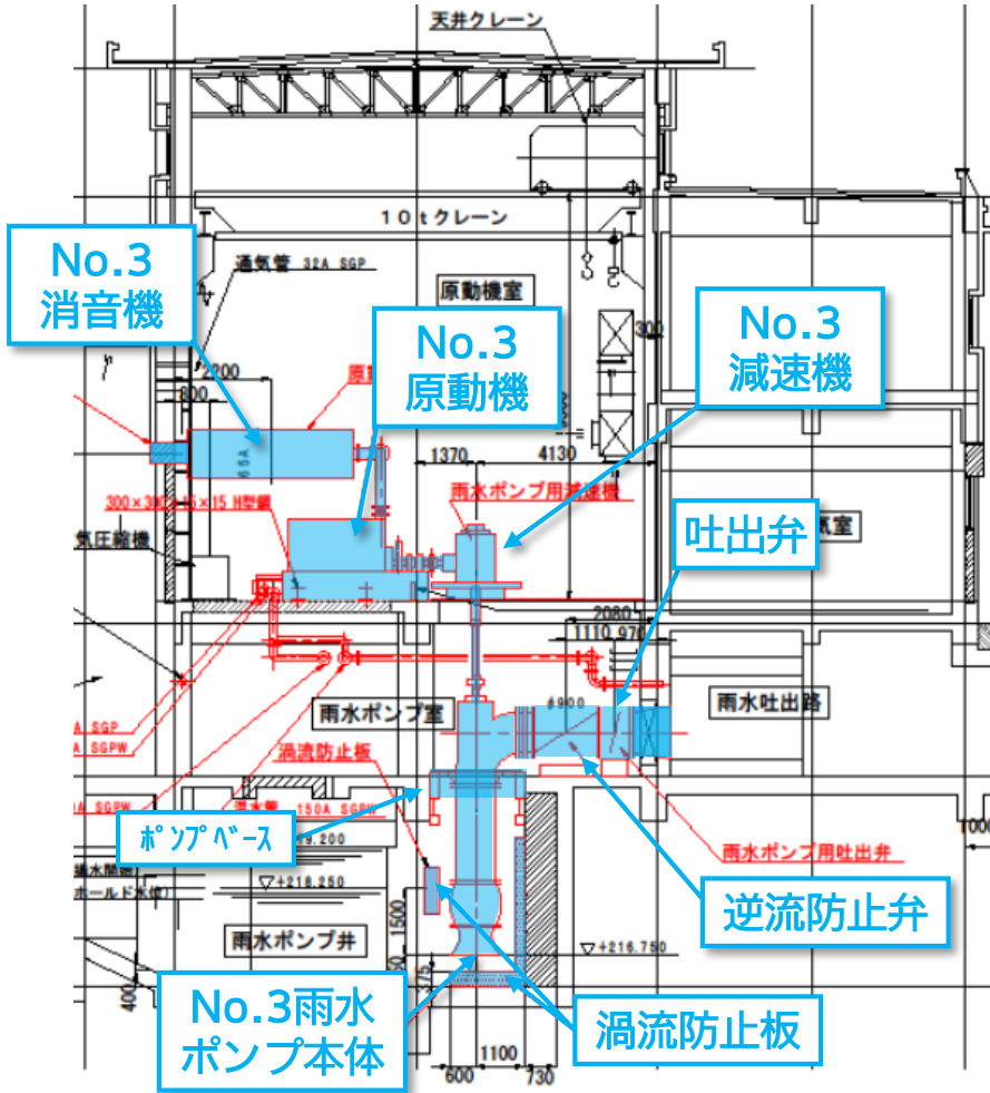
断面図(1階・地下1階・地下2階)
