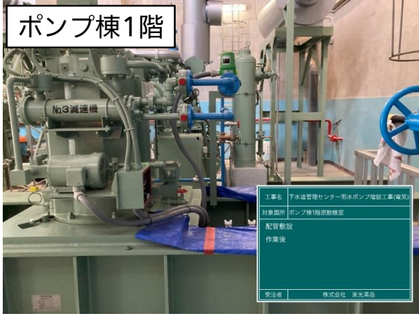
配管・配線(No.3減速機周辺)状況
