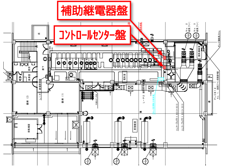
平面図(ポンプ棟2階)
