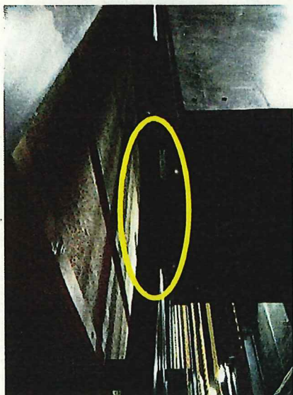
文化センター大ホール 吊り物レール破損
