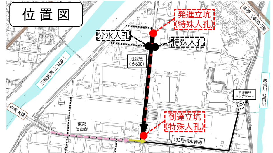
交通規制図 (発進立坑)
