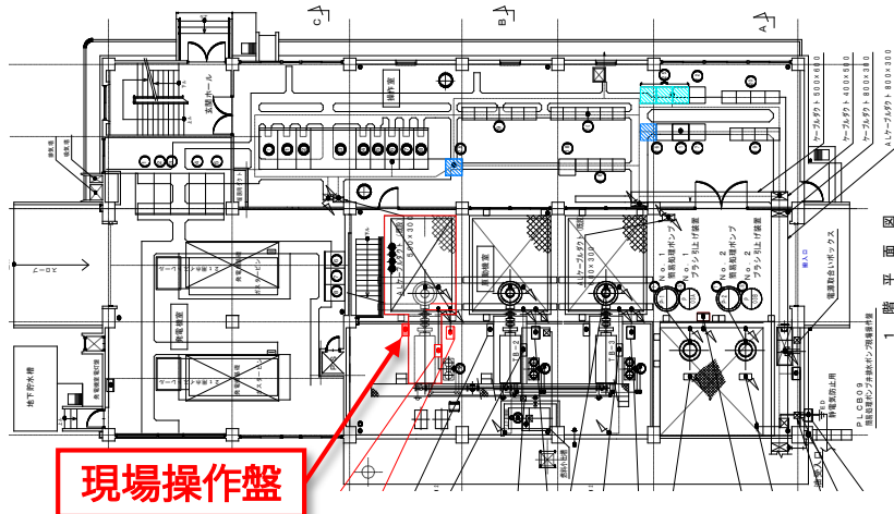
平面図(ポンプ棟1階)
