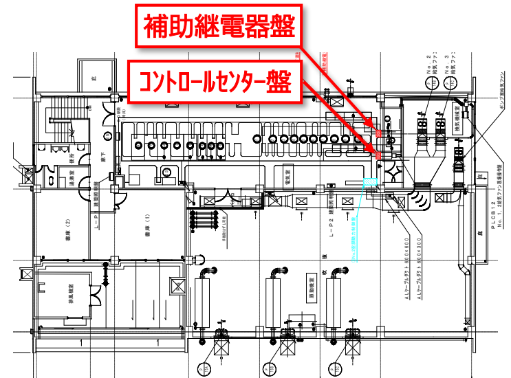
平面図(ポンプ棟2階)
