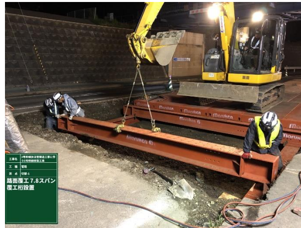
覆工板設置状況
