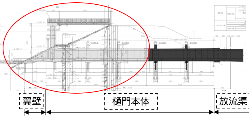
吐口樋門 一般図
