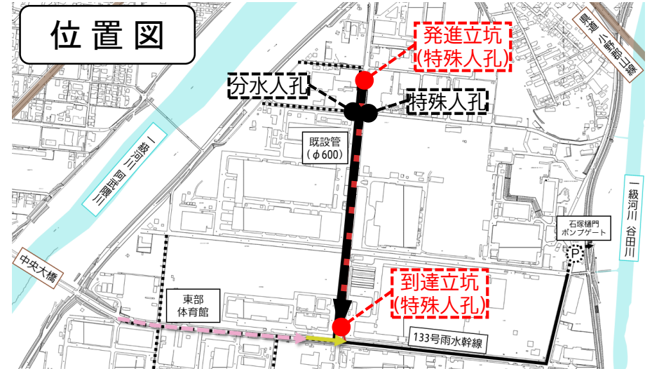
交通規制図 (発進立坑)
