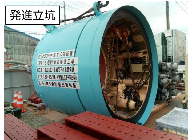
掘進機搬入状況
