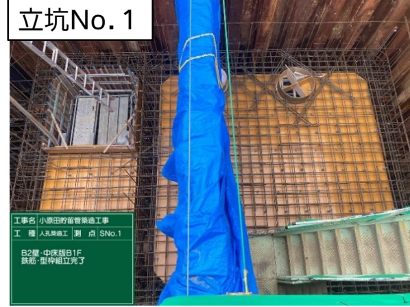
立坑No.1特殊人孔配筋・型枠組立
