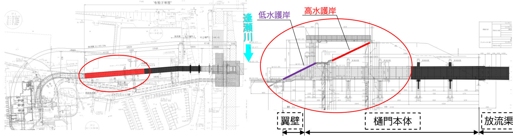
平面図（施工中放流渠部）
