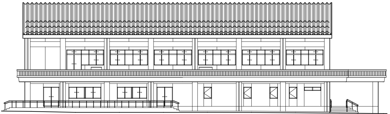
南側立面図
