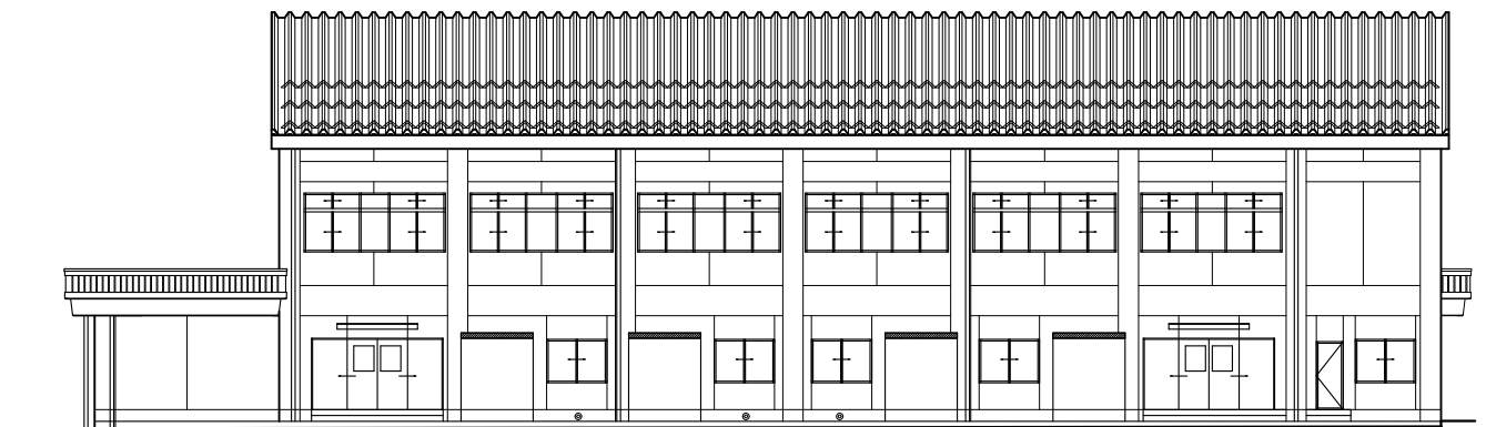
北側立面図
