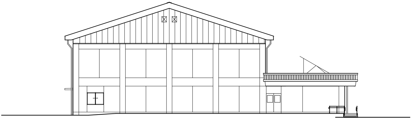
西側立面図
