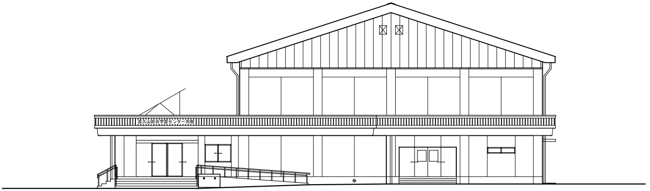
東側立面図
