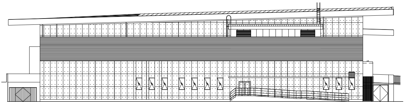
東側立面图
