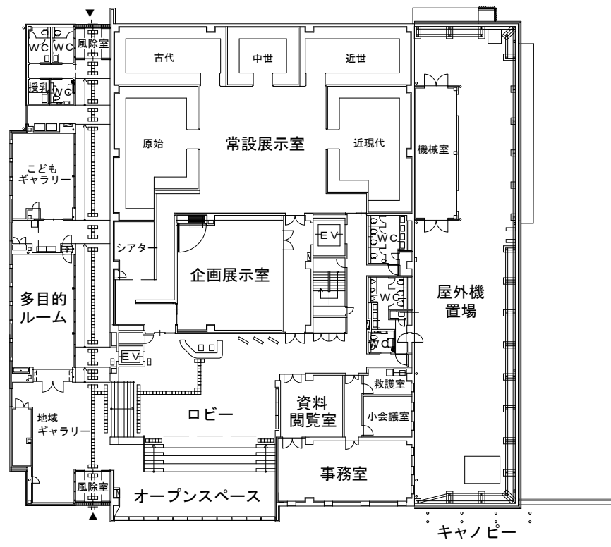
1階平面図
