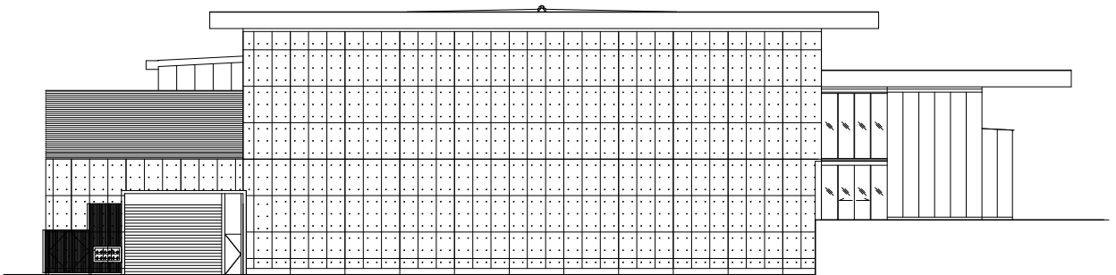
北側立面图
