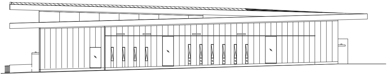
西側立面图
