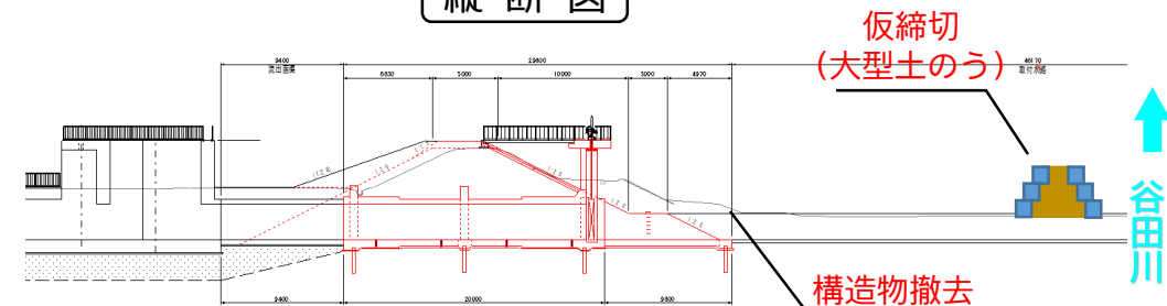
縦断図
