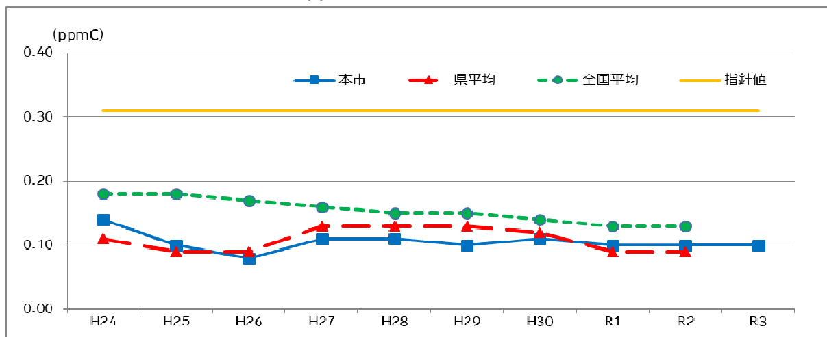
図 11 非メタン炭化水素濃度 (6 時～9 時における年平均値) の推移
