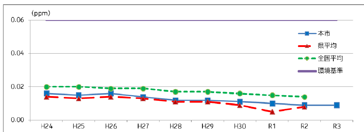
図 7 二酸化窒素濃度 (年平均値) の推移
