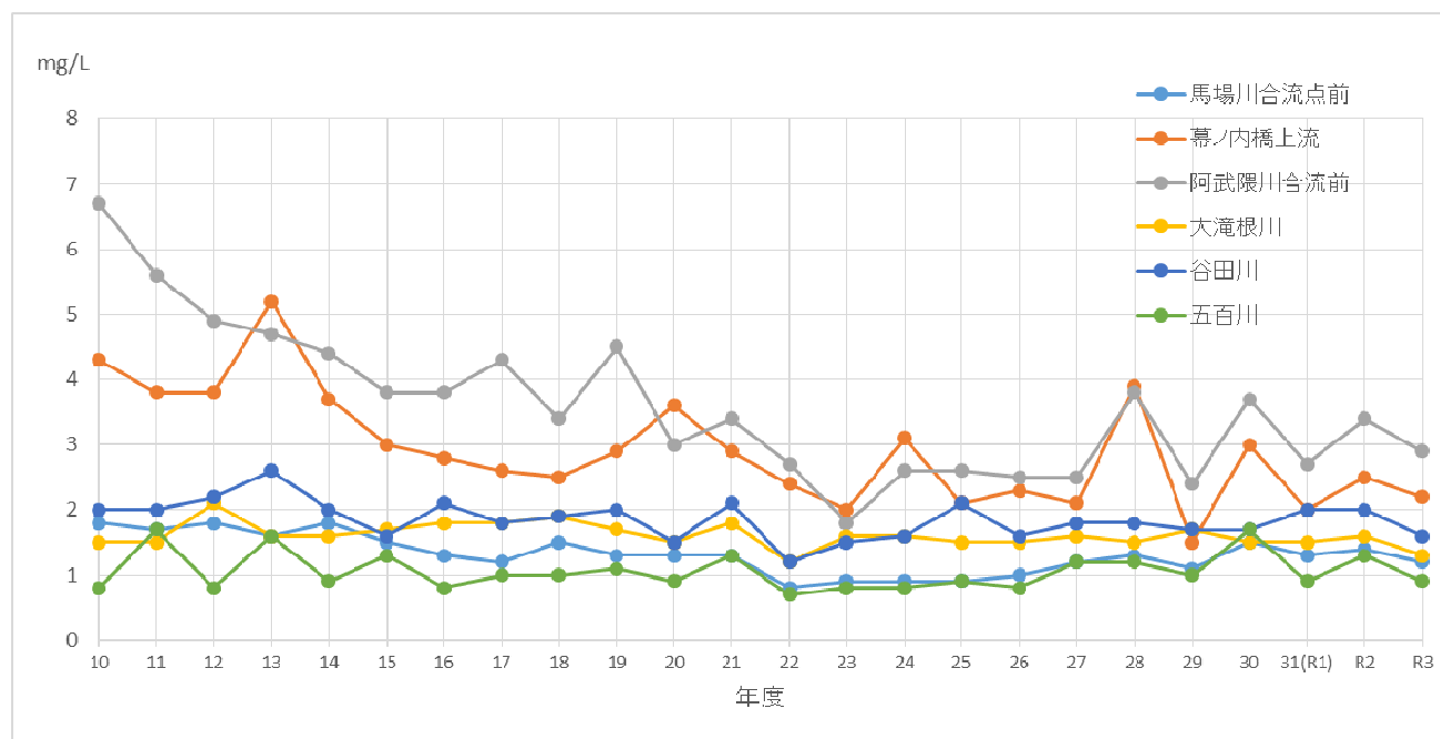
図1 河川のBOD値の推移
