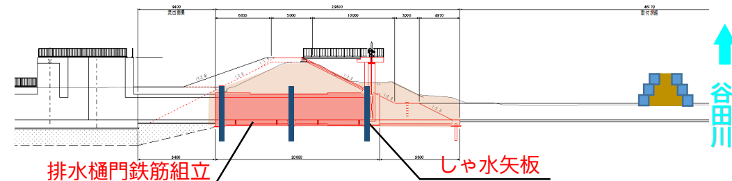
縦断図
