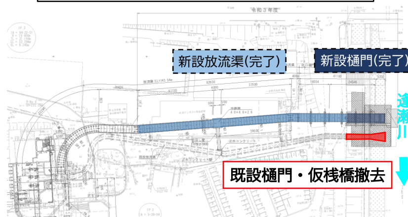
仮棧橋撤去状況
