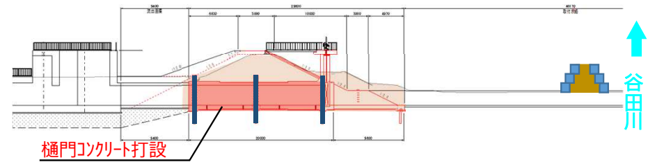
縦断図
