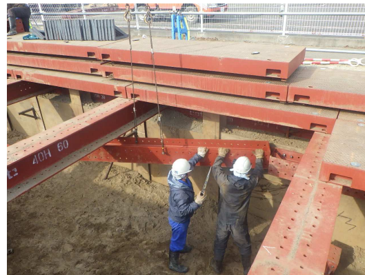
切梁・腹起し設置状況
