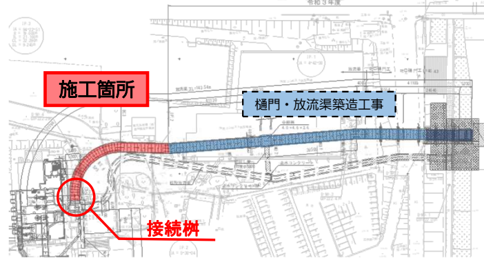
平面図
