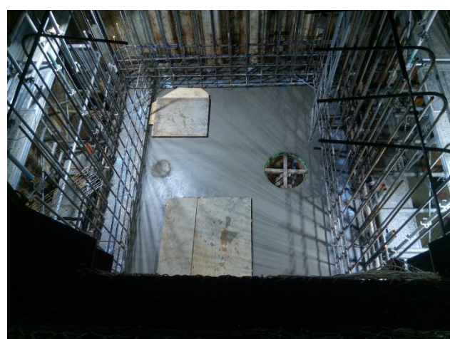
上段スラブ打設完了 (特殊人孔No.2)
