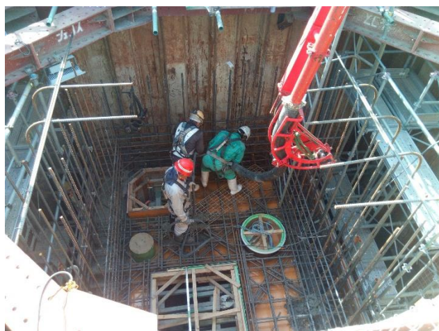
上段スラブ打設状況 (特殊人孔No.2)
