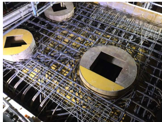
頂版鉄筋組立完了 (特殊人孔No.2)
