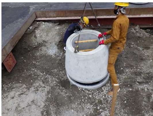
分水人孔②マンホール設置状況
