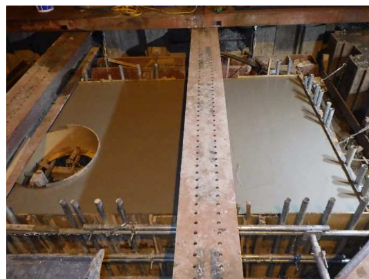
分水人孔③コンクリート打設完了
