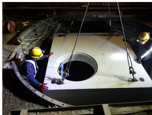
分水人孔③取込人孔頂版設置状況
